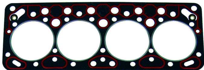
56108701 Ø 98,5 mm
