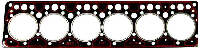
56149603 Ø 98,5 mm
